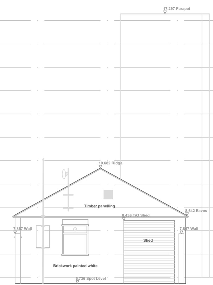
Elevation E5
